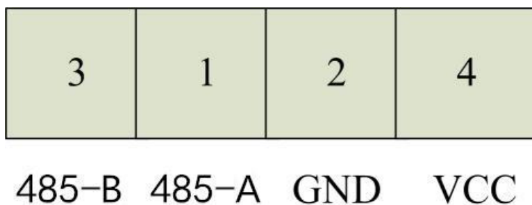
图 2.2 RS485 接线端子电气定义
