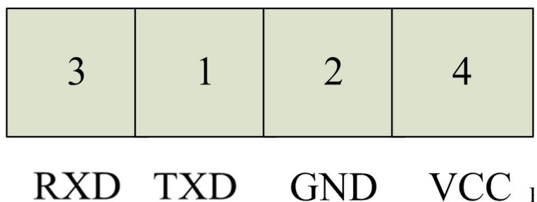
图 2.1 RS232 接线端子电气定义
